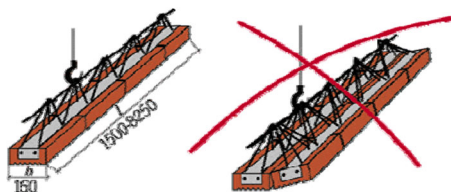
Obr. 9 Při manipulaci jeřábem lze manipulovat pouze s jedním zavěšeným nosníkem
