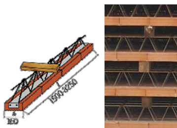
Obr. 8 Správná poloha umístění prokladů Obr. 7 Ukázka slohy stropních nosníků
